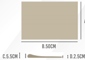
15 BORDE RECTO 50 1003502
