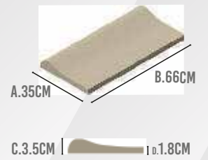
13 BORDE RECTO 66 1003502
